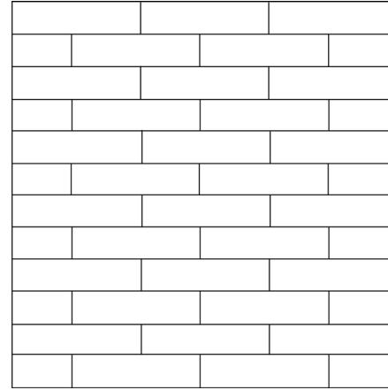
Halvforbandt vandret*
